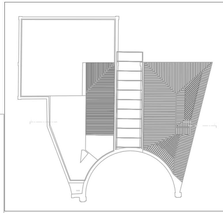
CÉU DE VÊRO PLANTA DA COBERTURA
