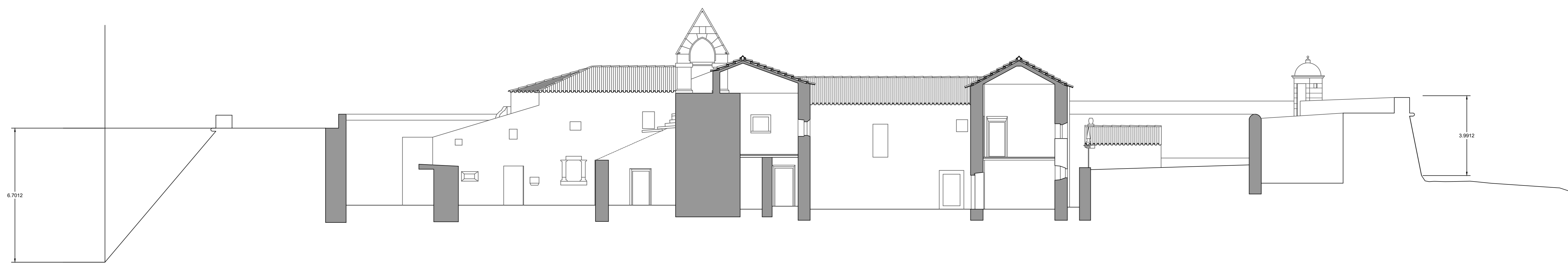
CORTE C-C'
