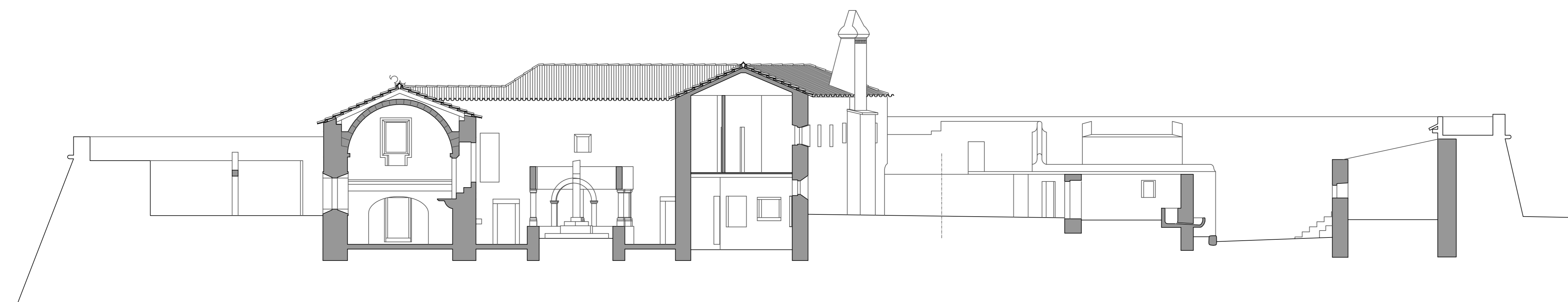
CORTE C-C'
