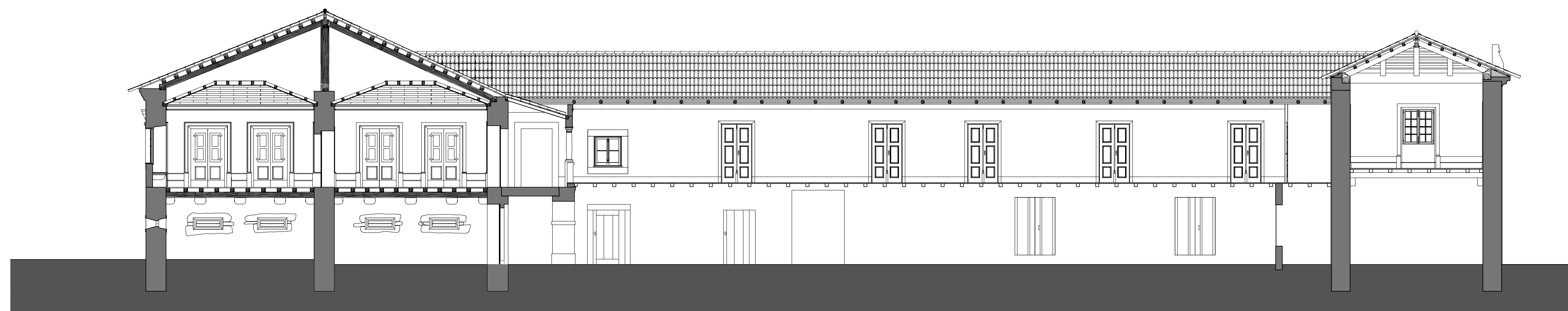
CORTE AA'
