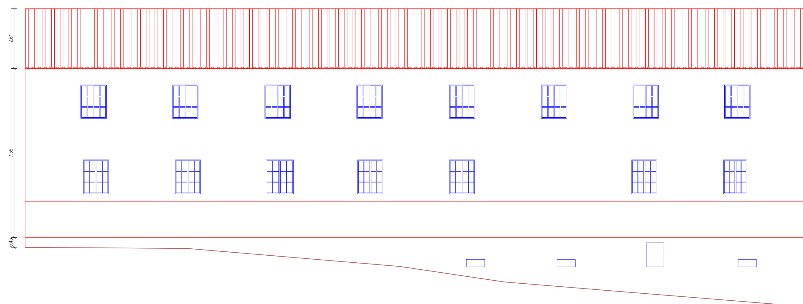
Alçado posterior
