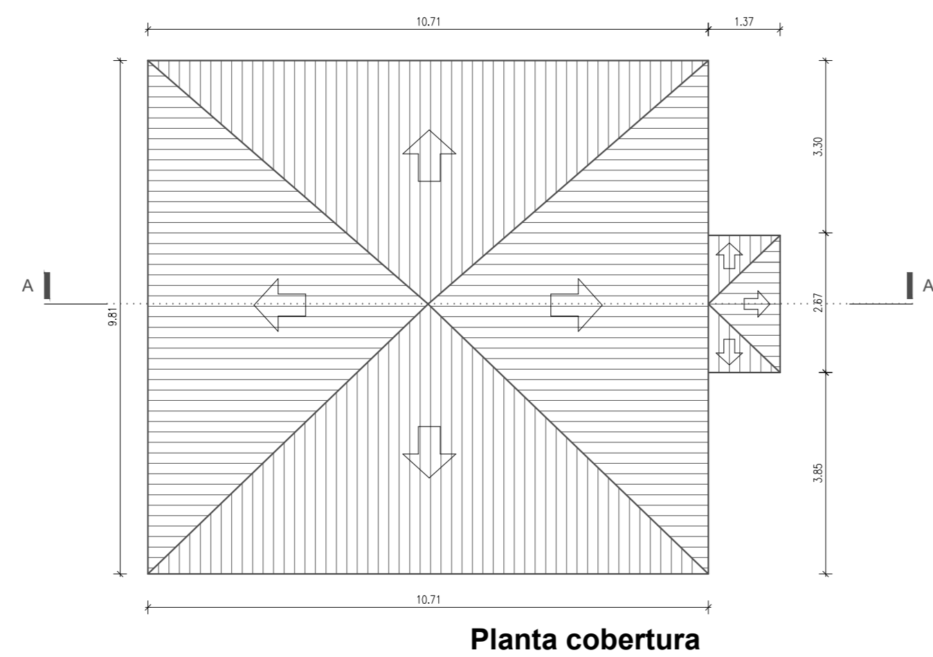
Planta cobertura
