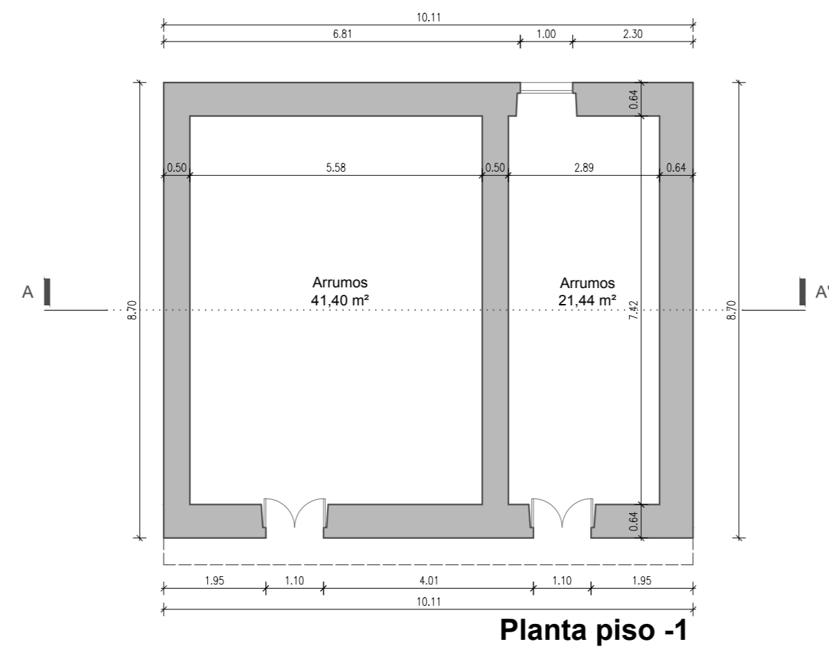
Planta piso -1
