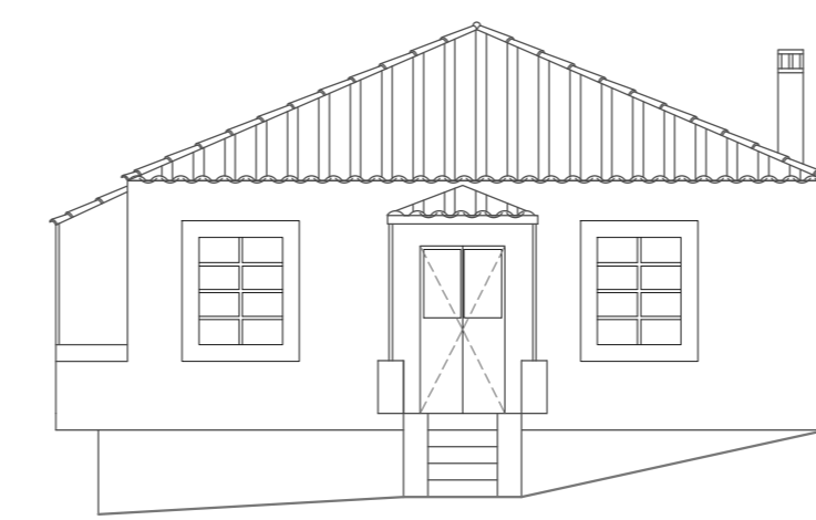
Alçado principal
