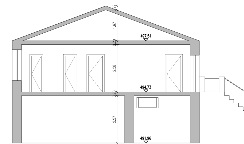
Corte AA'
