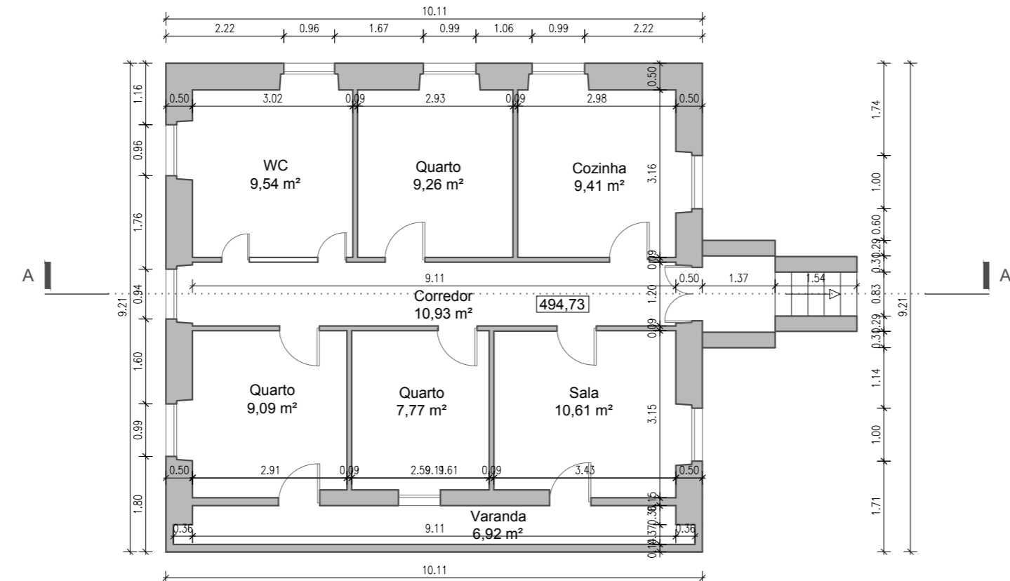
Planta piso 0
