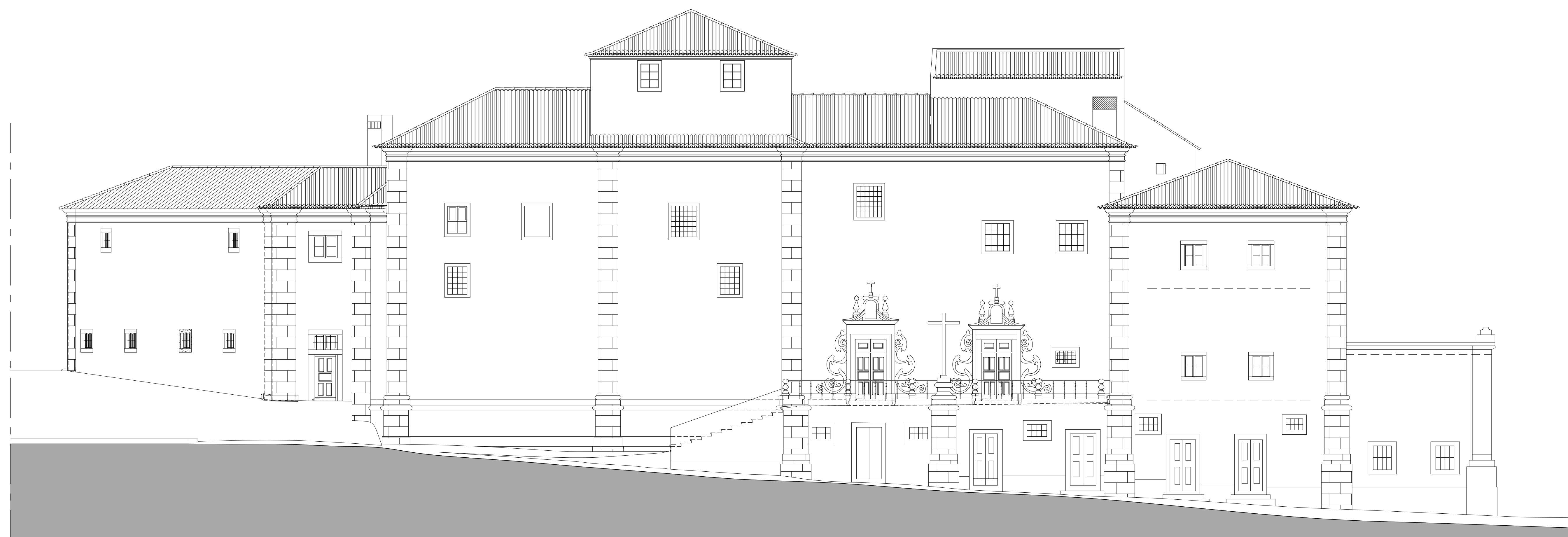
Alçado Oeste Esc. 1:100
