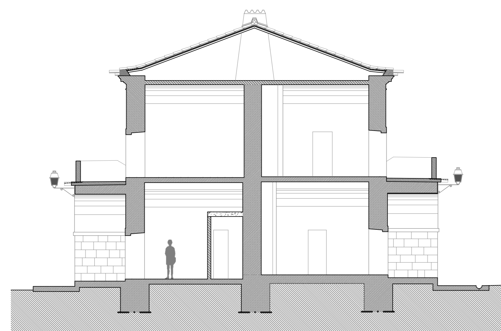
CORTE C-D
