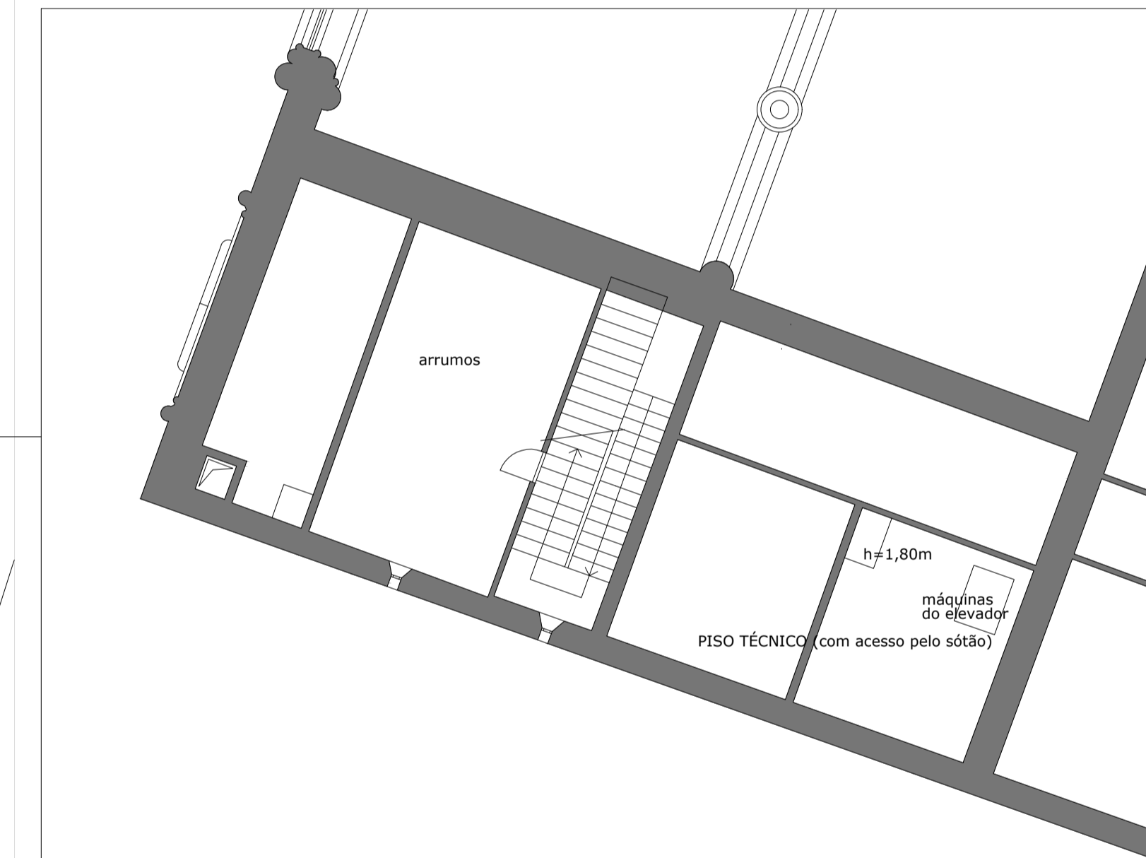
PISO INTERMÉDIO 94,56m 2
