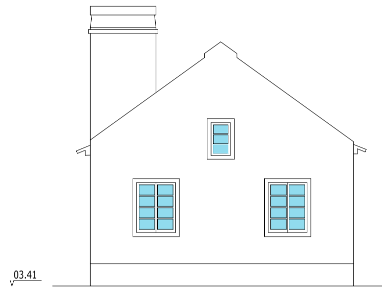
ALÇADO POENTE
