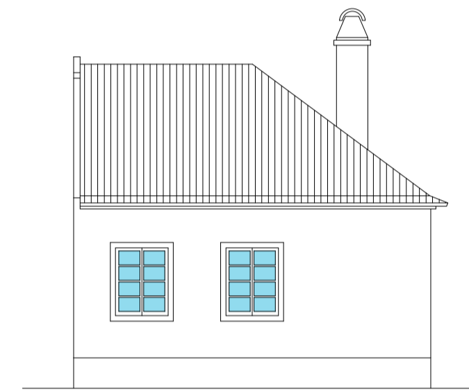
ALÇADO NORTE
