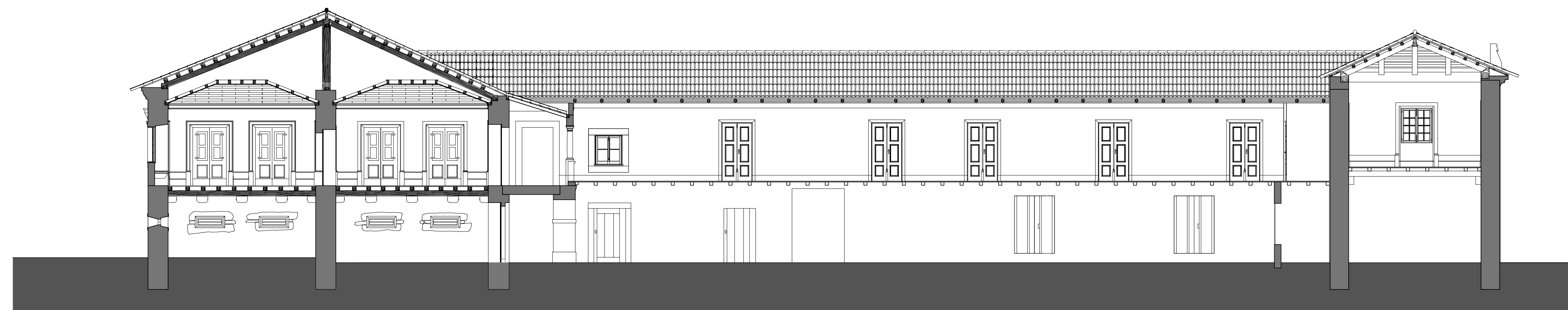
CORTE AA'
