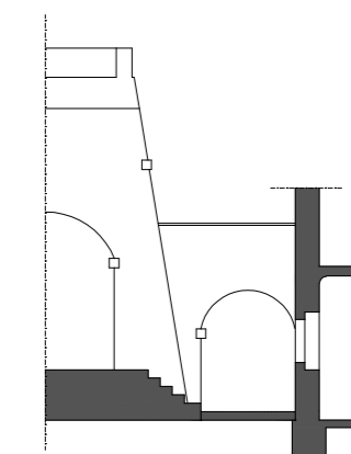
Corte GH
