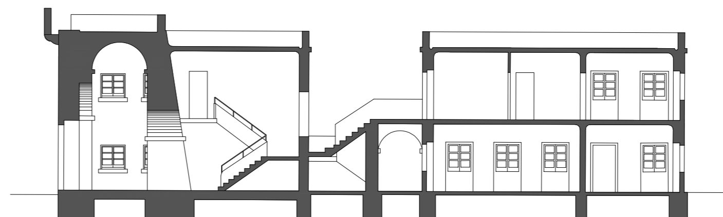
Corte CD
