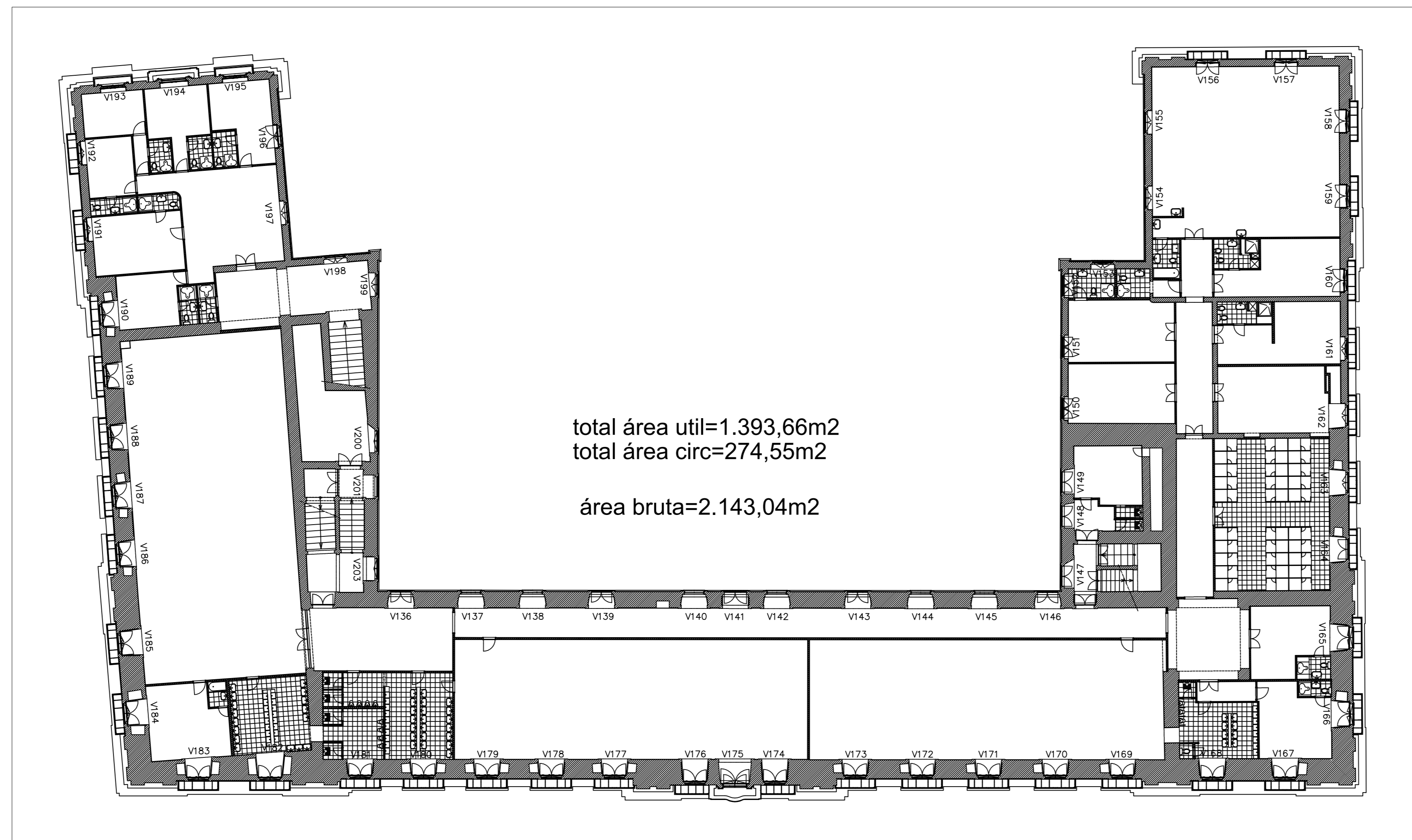
PLANTA DO 2.º ANDAR
