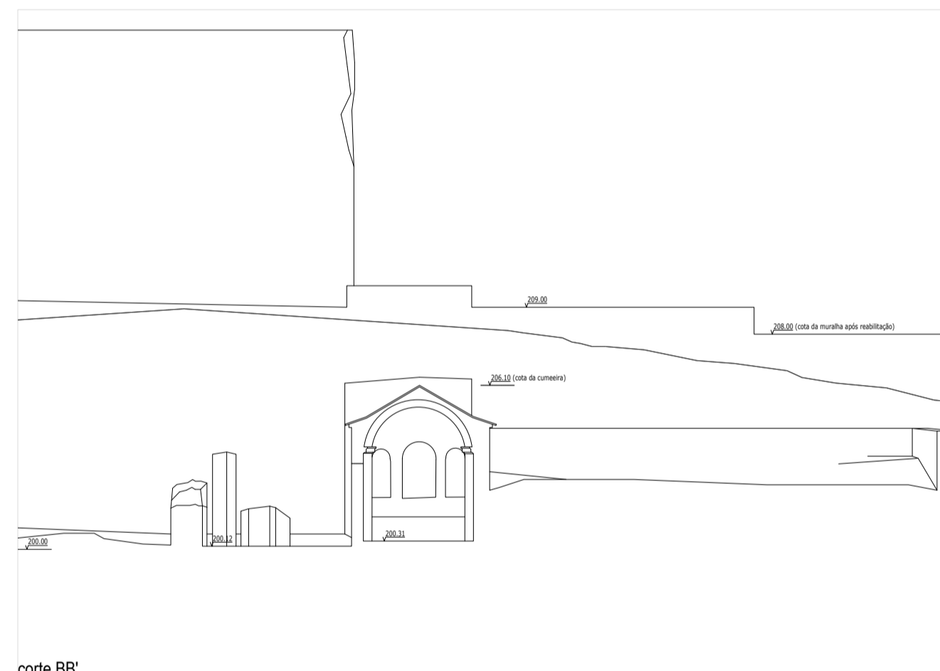
corte BB'
