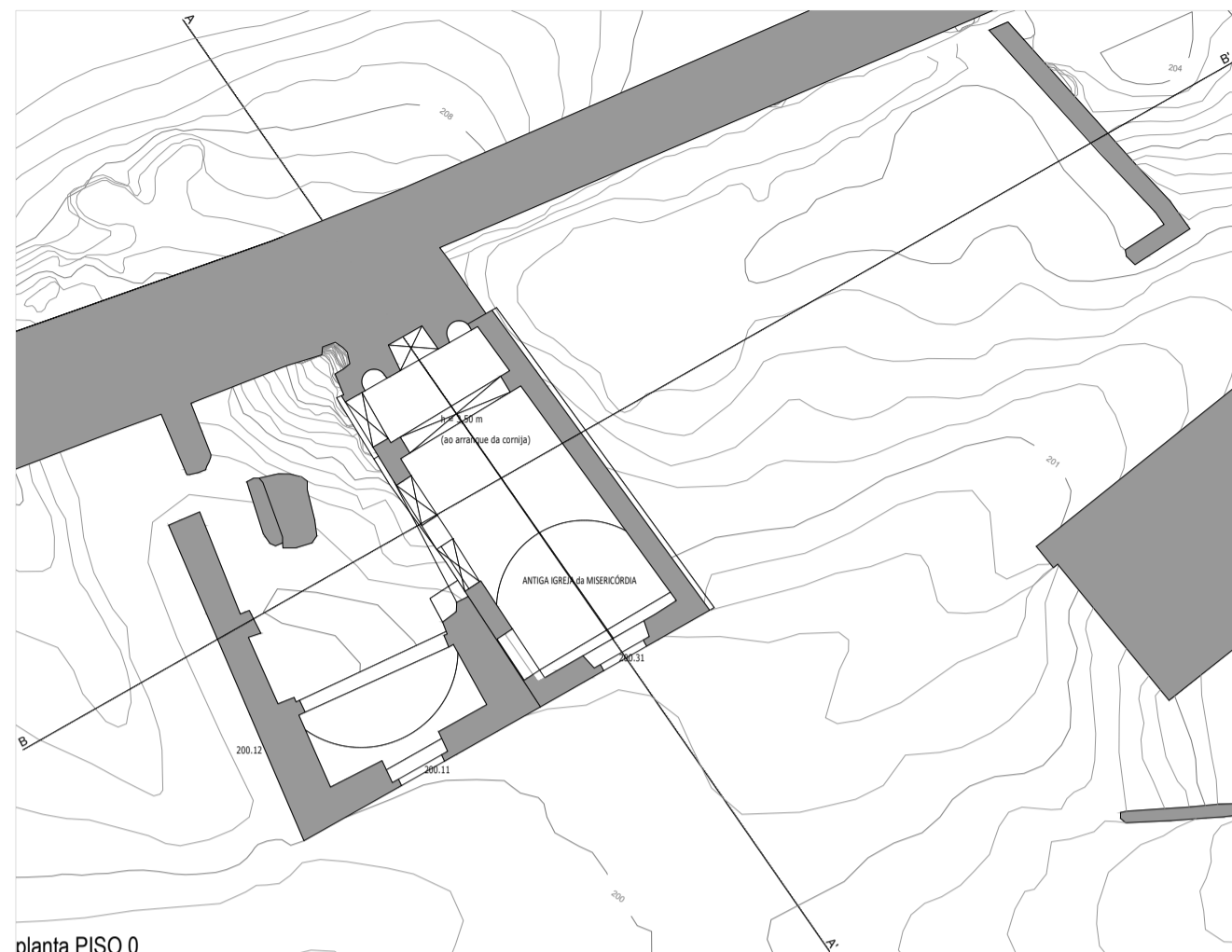
planta PISO 0
